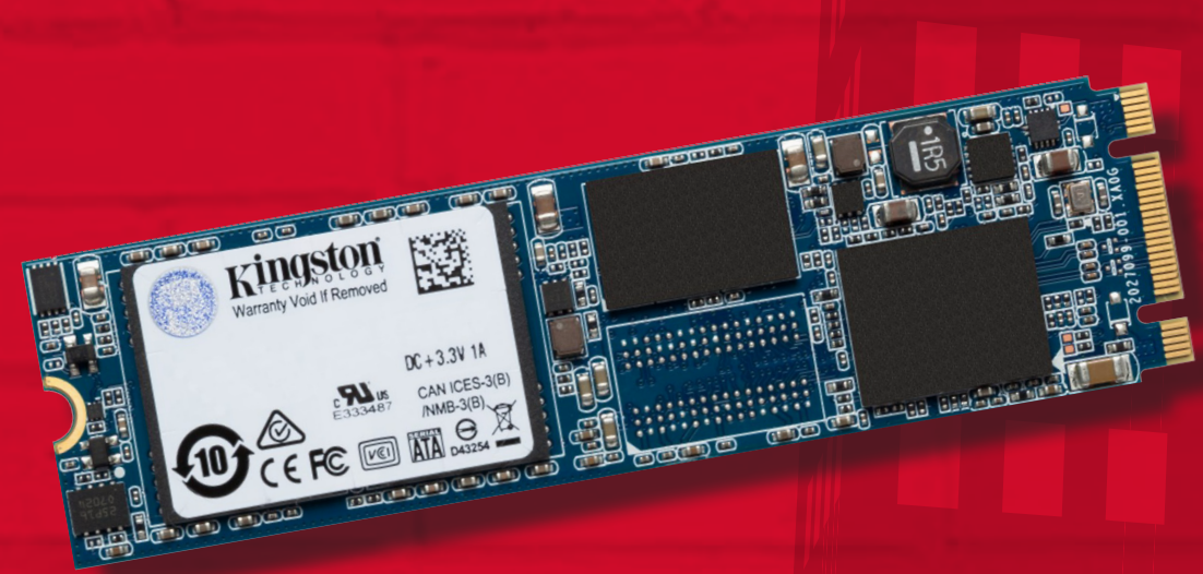
M.2 SSD
